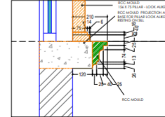
D11 DETAIL SCALE: 1:10
