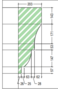
MD1 MOULDING DETAIL SCALE: 1:5
