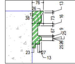
MD2 MOULDING DETAIL SCALE: 1:5
